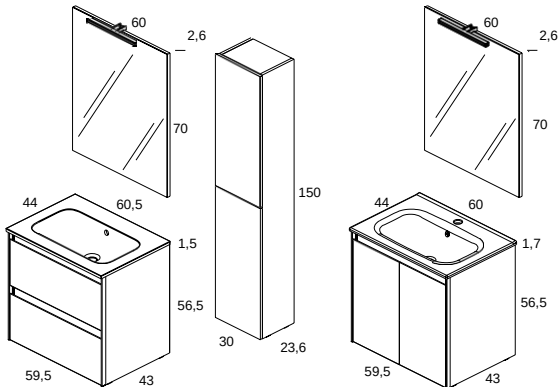
LOOK C0071313 Conjunto 60 F-44 · 2P
