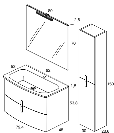
Nuevo lavabo cerámico TREND
