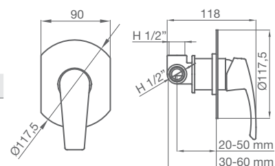
MECANISMO EMPOTRABLE
