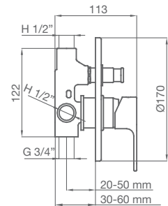
MECANISMO EMPOTRABLE
