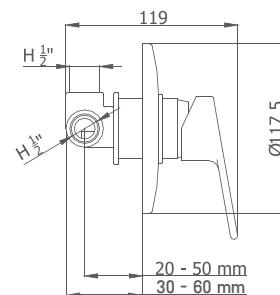
MECANISMO EMPOTRABLE
