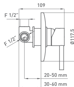
MECANISMO EMPOTRABLE
