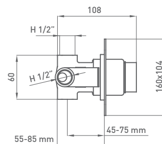
MECANISMO EMPOTRABLE CON MANETAS
