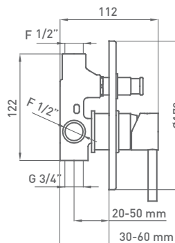
MECANISMO EMPOTRABLE
