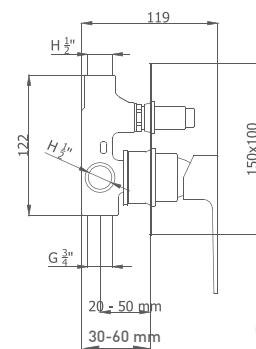
MECANISMO EMPOTRABLE
