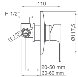
MECANISMO EMPOTRABLE
