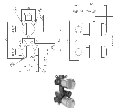
MECANISMO EMPOTRABLE CON MANETAS
