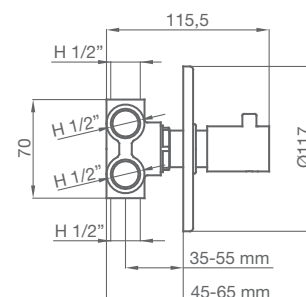
MECANISMO EMPOTRABLE
