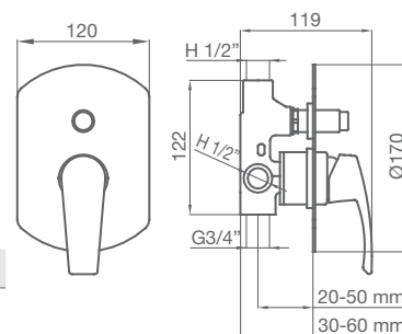
MECANISMO EMPOTRABLE
