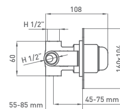
MECANISMO EMPOTRABLE CON MANETA
