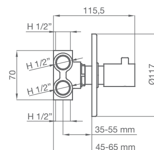
MECANISMO EMPOTRABLE
