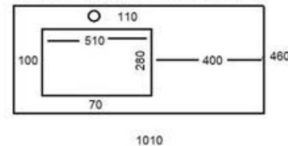
LAVABO DE 1010X460 1 SENO IZQUIERDO
