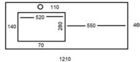
LAVABO DE 1210X460 1 SENO IZQUIERDO
