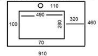
LAVABO DE 910X460 1 SENO IZQUIERDO
