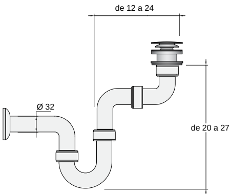
Juego sifón reducido más válvula clicker 19366
