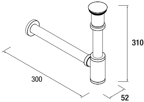
Sifón SMART con válvula clicker 23033
