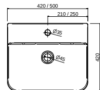
Lavabo de posar TENTO 500 porcelana blanca sin sifón ni desagüe 500 x 420 x 130 mm
