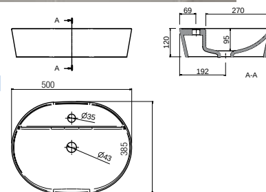
Lavabo de posar VARMEGA 515 porcelana blanca sin sifón ni desagüe 500 x 385 x 120 mm
