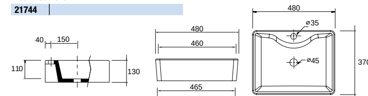
Lavabo de posar EMOTION porcelana blanca sin sifón ni desagüe 480 x 130 x 370 mm
