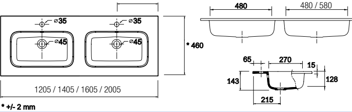
Lavabo SOFIA 1605 doble MineralMarmo sin sifón ni desagüe clicker 1605 x 15 x 460
