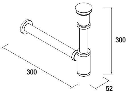
Sifón SMART con válvula abierta 23032
