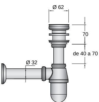
Sifón con desagüe latón cromado 9699
