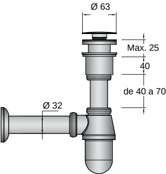
Sifón válvula abierta con desagüe latón cromado 16994
