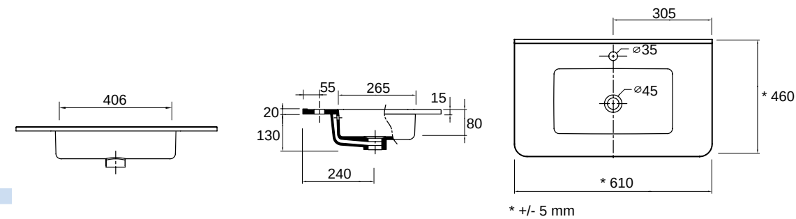
Lavabo ARADIA 610 porcelana blanca sin sifón ni desagüe clicker 610 x 20 x 460 mm
