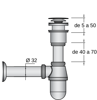
Sifón con desagüe clicker latón cromado 13663
